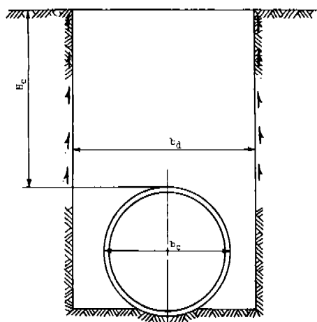
Fig. 1-1 Ditch conduit
