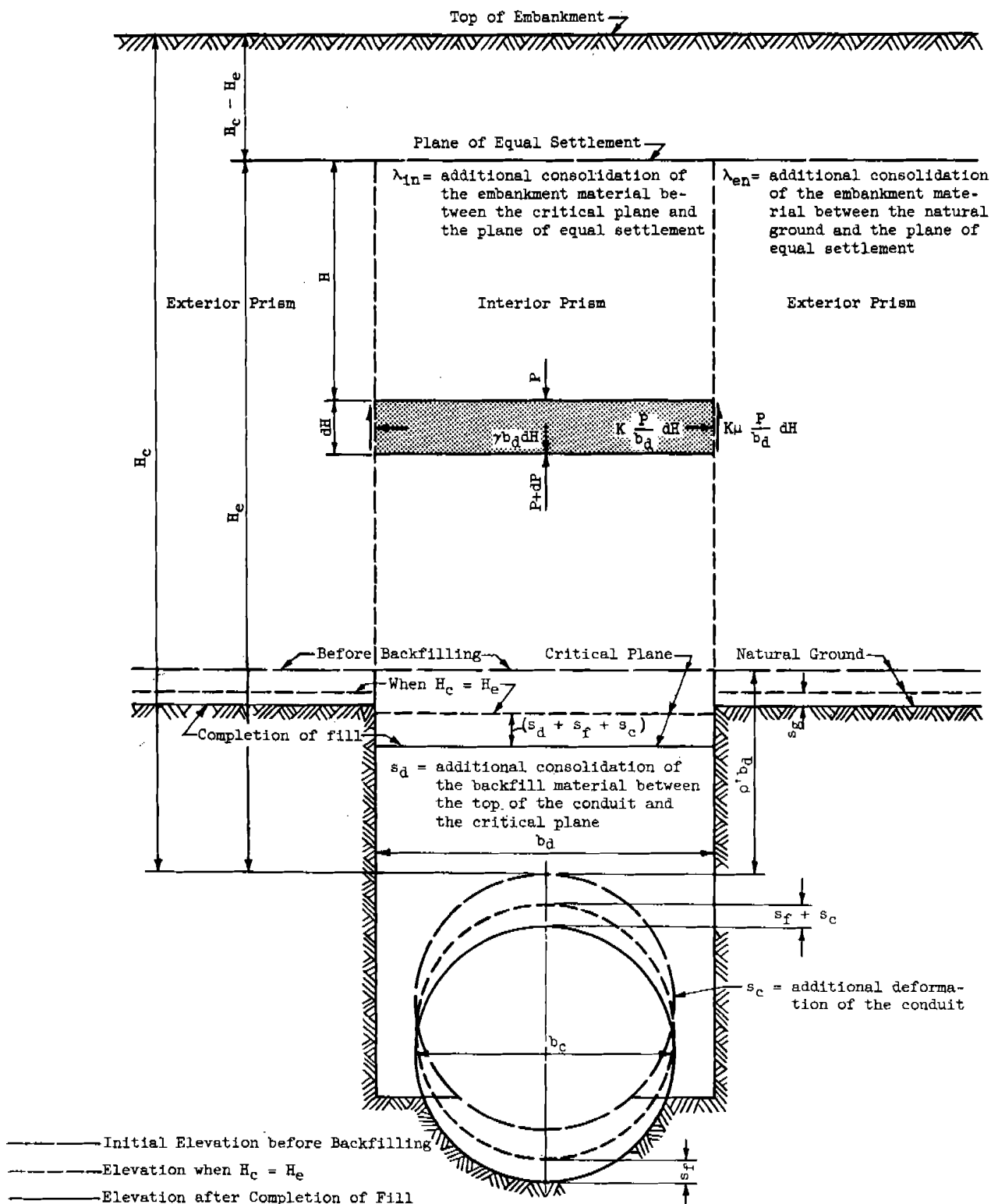
Fig. A-6 Negative projecting conduit
